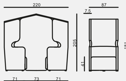
Dimensioni cellula acustica a 2 posti assemblata
