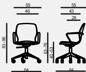
Box gross weight 14,4 kg – Vol. box 0,37 m³
